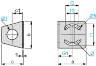
尺寸 (毫米)
