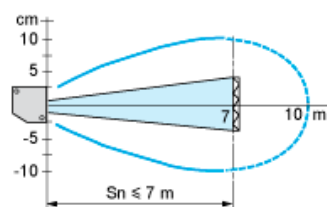
带反光板 XUZC50
