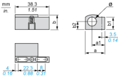
尺寸 (毫米)
